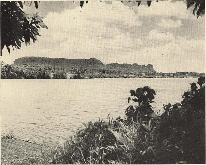
FIGURE 3.—Jokaj Rock.
